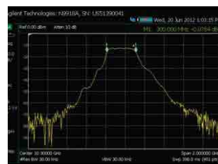
Следящий генератор
