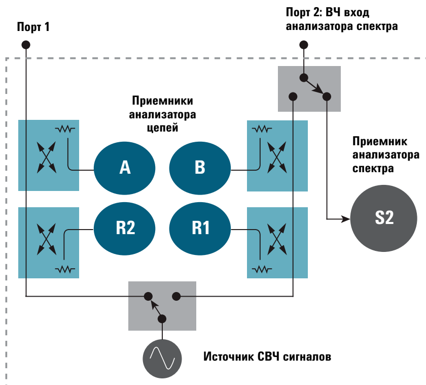
Архитектура СВЧ-анализаторов FieldFox
