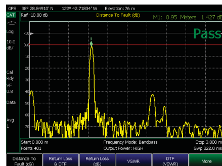
Анализатор антенно-фидерных устройств
