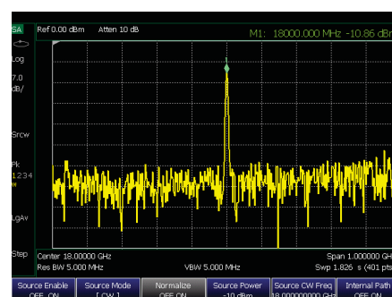
Использование внутреннего источника СВЧ сигналов для испытания ретранслятора
