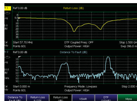
Окно измерения потерь на отражение и расстояния до неоднородности
