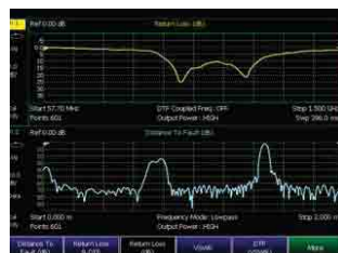
Анализ антенно-фидерных устройств
